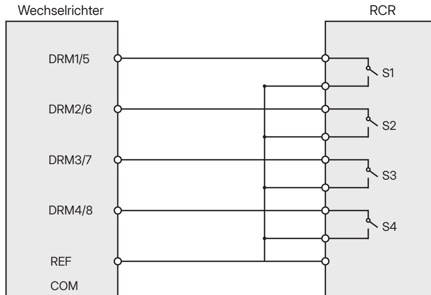
Abbildung 7-5 RCR-Anschluss
