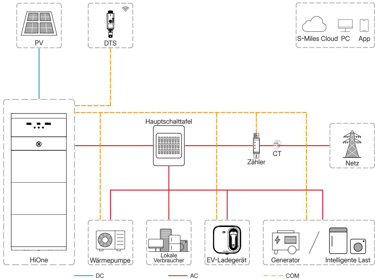
Abbildung 5-1 Grundsystem
