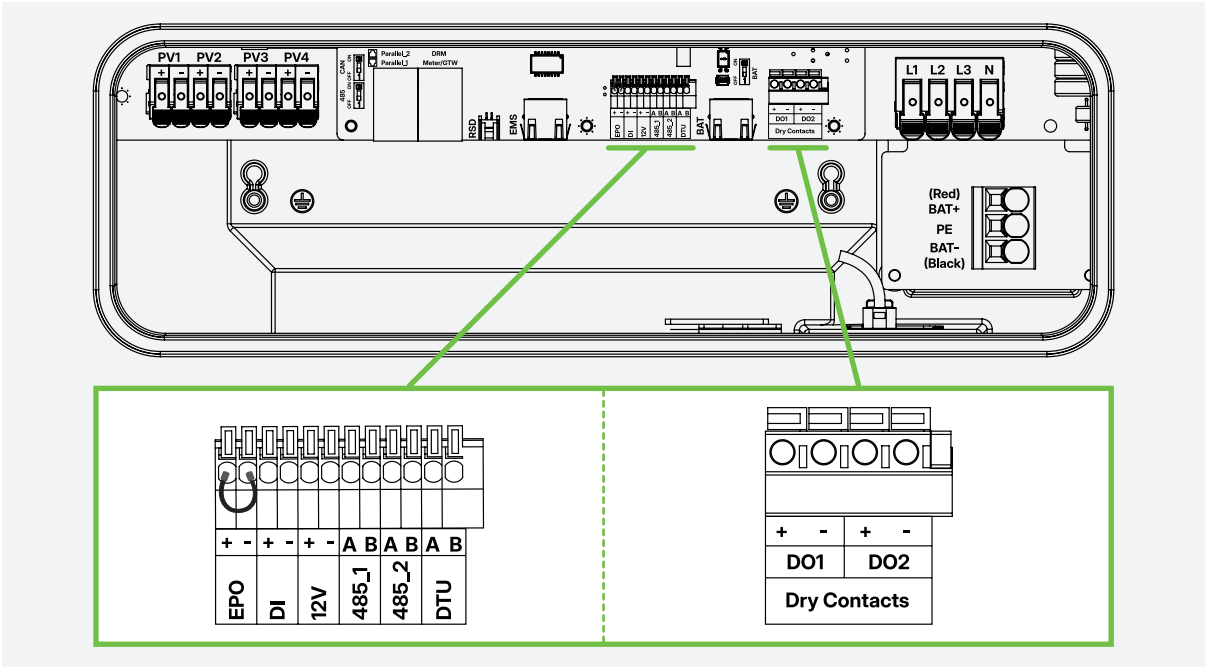
Abbildung 7-6 COM2-Übersicht
