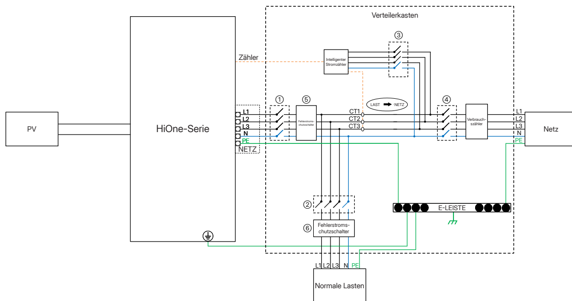
Abbildung 7-1 Grundsystem
