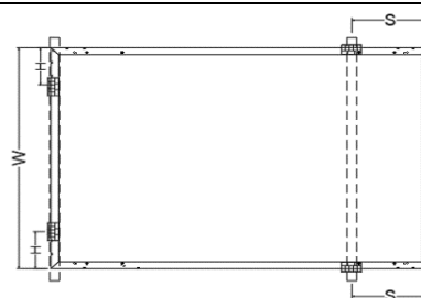
Abbildung 11 Klemme-F
